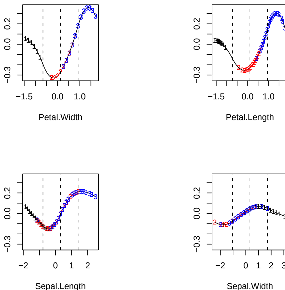
Figure 8 : La décomposition de type ANOVA pour t^2 , les variables sont ordonnées par ordre décroissant d'influence, de la gauche vers la droite et du haut vers le bas, selon l'étendue des valeurs sur l'axe vertical. Le codage des observations : setosa (1), versicolor (2), virginica (3). Les verticales en pointillés indiquent la position des noeuds.
