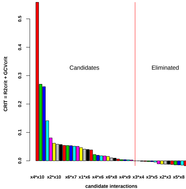
Figure 1 : Classement des interactions candidates à l'entrée dans le modèle de la réponse y^4 des données de polymérisation. L'interaction x^4 * x^{10} arrive en tête. C'est la seule acceptée au seuil de 20% avec un gain du GCV de 52.18%.
