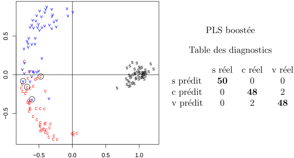
Figure 6 : À gauche, le nuage des observations des Iris setosa (s), versicolor (c) et virginica (v), dans le plan (t^1, t^2) du modèle PLSS. Les individus mal affectés à leurs groupes réels sont entourés d’un cercle. À droite, les diagnostics d’affectation des observations, les individus biens classés sont en gras.
