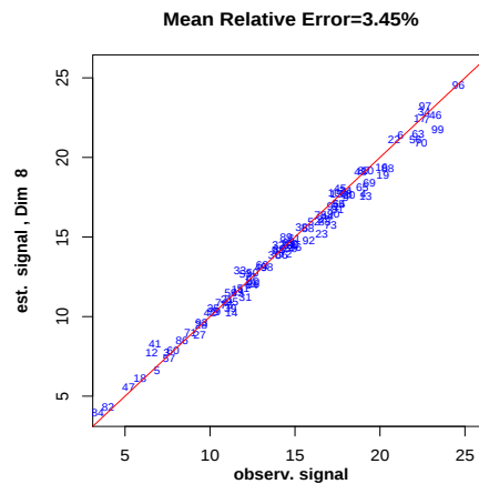
Figure 2 : Prédiction MAPLSS à 8 dimensions sur l'échantillon test des données simulées : valeurs prédites contre valeurs du signal.
