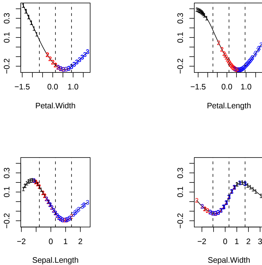
Figure 7 : La décomposition de type ANOVA pour t^1 , les variables sont ordonnées par ordre décroissant d'influence, de la gauche vers la droite et du haut vers le bas, selon l'étendue des valeurs sur l'axe vertical. Le codage des observations : setosa (1), versicolor (2), virginica (3). Les verticales en pointillés indiquent la position des noeuds.
