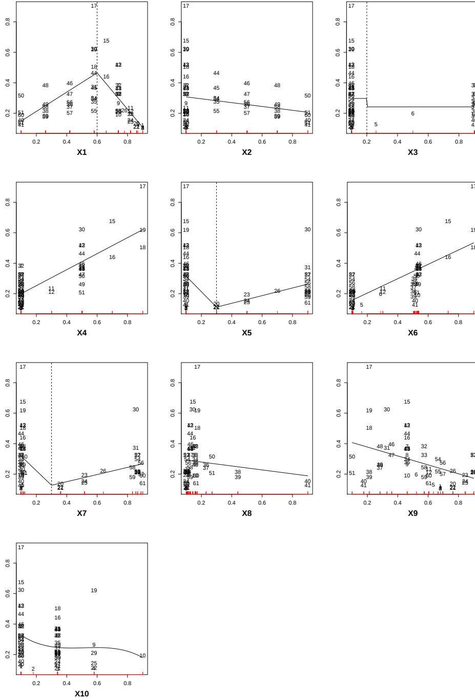
Figure 3 : Les 10 nuages de points (x^j, y^4)_{j=1,10} du jeu de données "chemdata", lissés par des splines aux moindres carrés. Les mêmes degrés et nœuds, repérés ici par les verticales en pointillés, sont utilisés dans PLSS et MAPLSS pour la modélisation des quatre réponses y^1, \dots, y^4 .
