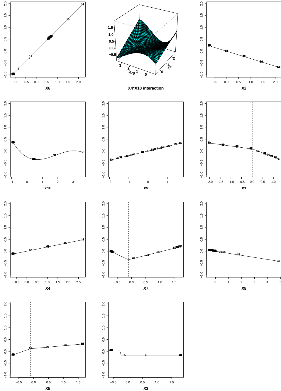
Figure 4 : La décomposition de type ANOVA de y^4 . Classement décroissant, de gauche à droite et de haut en bas, selon l'étendue des valeurs sur l'axe vertical.
