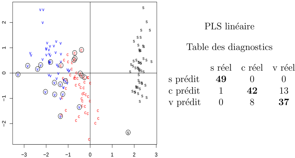
Figure 5 : À gauche, le nuage des observations des Iris setosa (s), versicolor (c) et virginica (v), dans le plan (t^1, t^2) de PLS linéaire. Les individus mal affectés à leurs groupes réels sont entourés d'un cercle. À droite, les diagnostics d'affectation des observations, les individus bien classés sont en gras.
